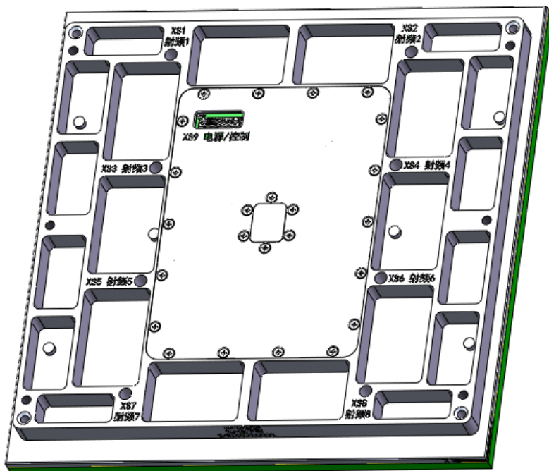
图 1 Ku 单波束接收子阵实物图
