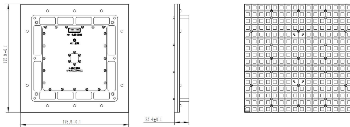
图 2 Ku 单波束接收子阵结构尺寸图
